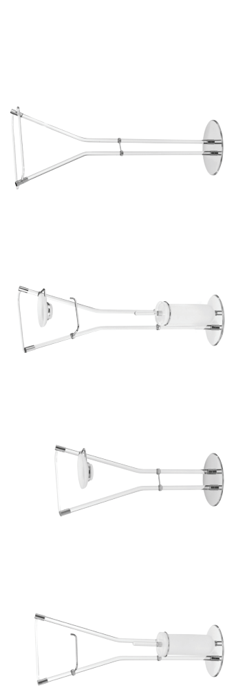
BASE CROMMUCHRONE BASE 793 Piantana wc Toilet stand Base Ø 205 L. 280 H. 710 mm 794 Piantana bidet Bidet stand Base Ø 205 L. 280 H. 620 mm
