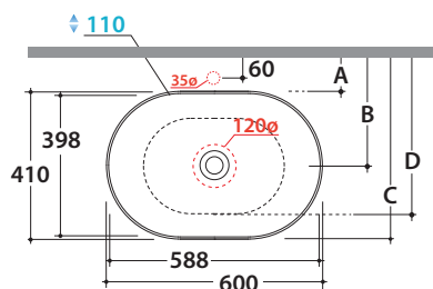
Installazione da appoggio / Sit-on installation
