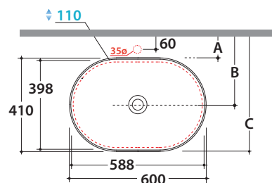
Installazione ad incasso / Recessed installation
