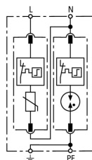
Schema di principio DG M TT 2P 275
